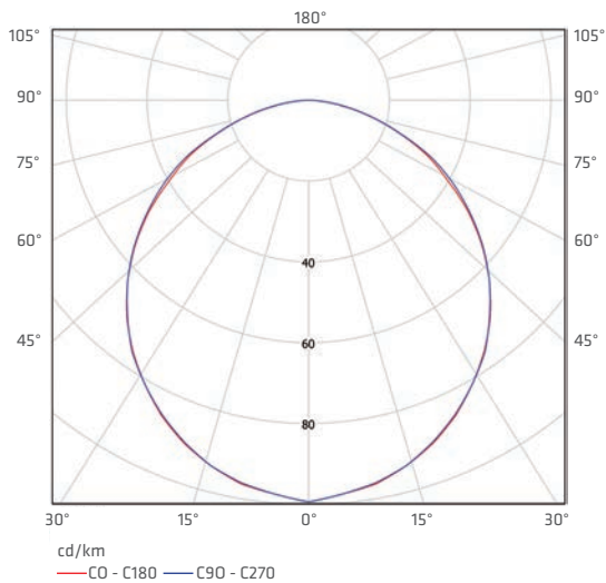
GLO 9x1W
